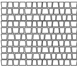
Schemat ułożenia elementów na palecie
