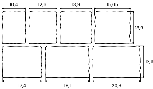
Schemat ułożenia elementów na palecie
