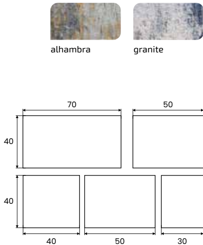
Schemat ułożenia elementów na palecie
