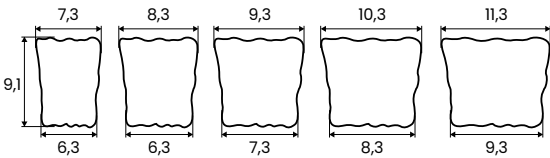
Schemat ułożenia elementów na palecie
