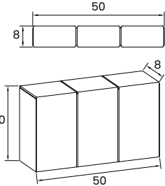
Schemat ułożenia elementów na palecie
