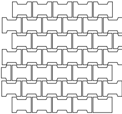
Schemat ułożenia elementów na palecie
