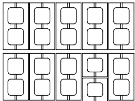
Schemat ułożenia elementów na palecie
