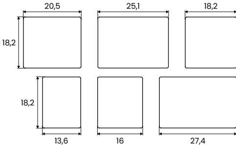
Schemat ułożenia elementów na palecie
