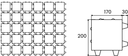
Schemat ułożenia elementów na palecie
