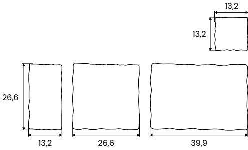
Schemat ułożenia elementów na palecie
